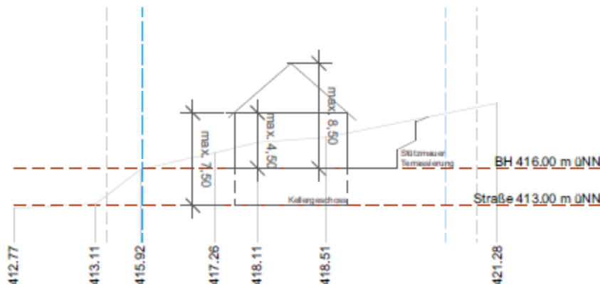
Beispielschnitt – Schnitt 10 (Lage siehe Planzeichnung) – ohne Maßstab
