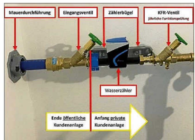
Wasserzähleranlage.
