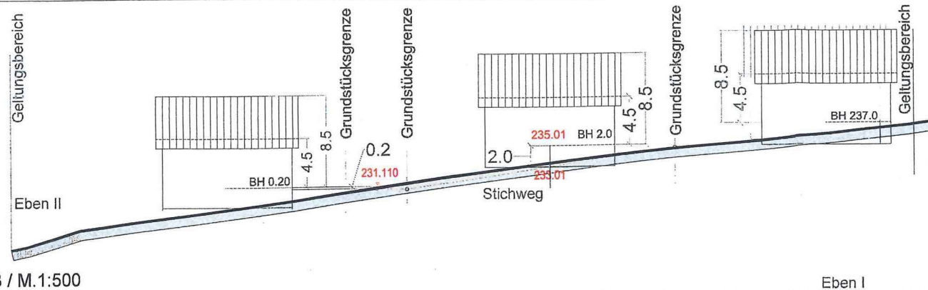
Systemschnitt 2 / M.1:500
