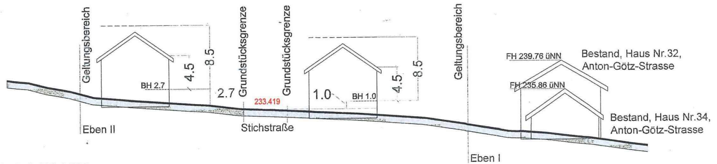
Systemschnitt 2 / M.1:500
