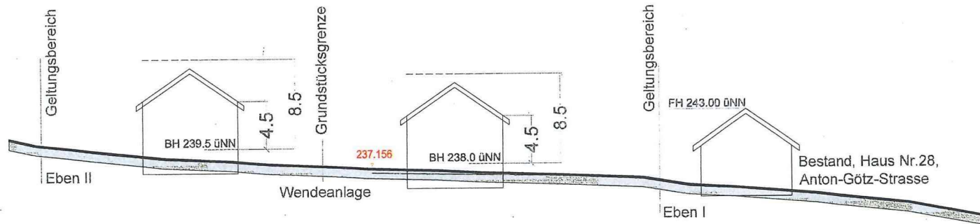
Systemschnitt 1 / M.1:500
